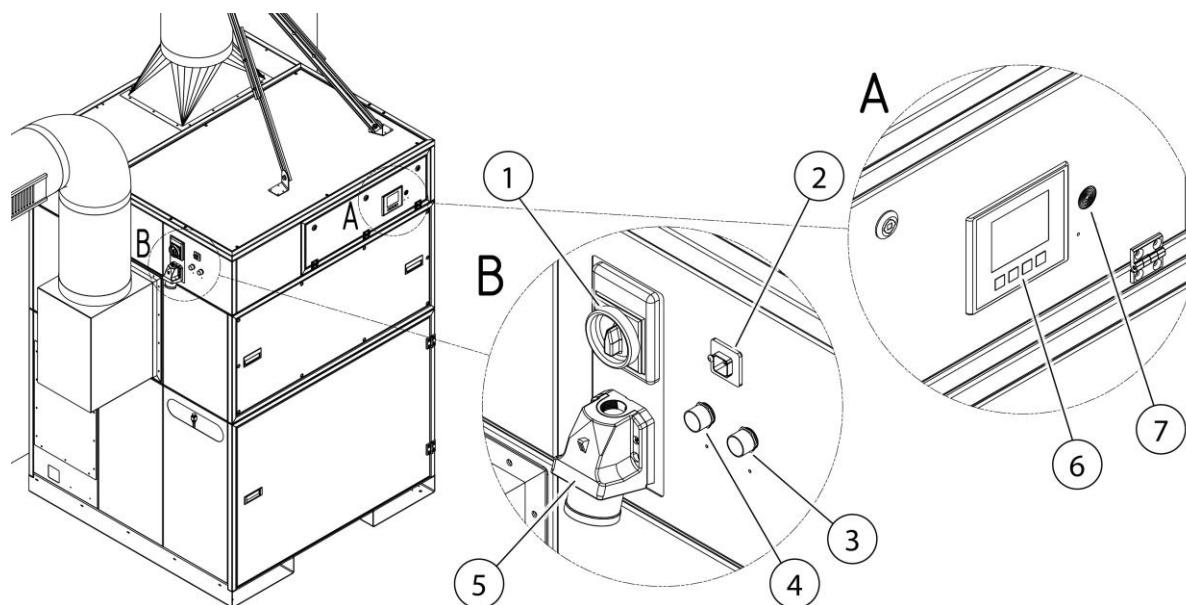
Fig. 7 : Panneau de raccordement et élément de commande
