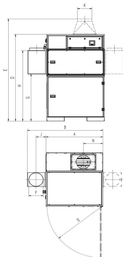
Fig. 54 : Fiche dimensionnelle 998701372 (998800407, 998800461)
