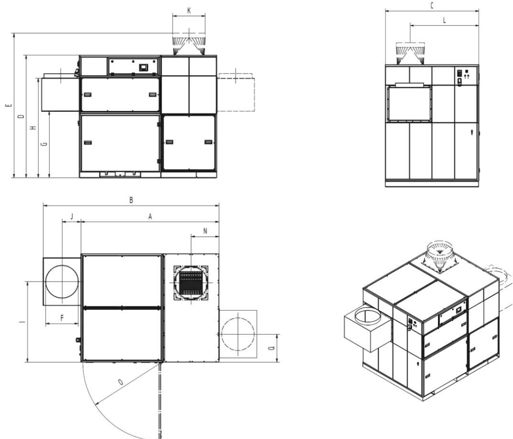
Fig. 56 : Fiche dimensionnelle 998701370 (998800414, 998800463)
