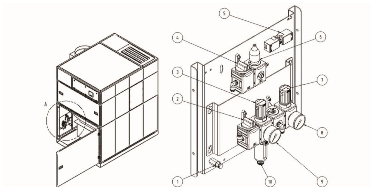
Fig. 10 : Unité d'air comprimé
